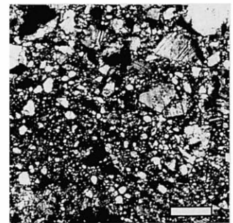
cataclasite (scale bar : 2mm)
