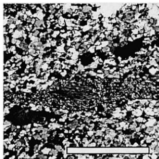
mylonite (scale bar : 2mm)
